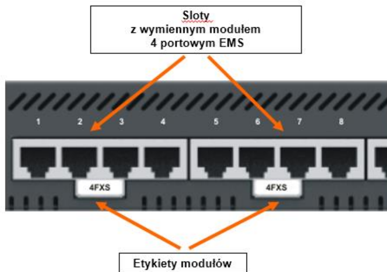
Ilustracja 4.18.: NCP-GWS – wersja z modułami 4 portowymi
