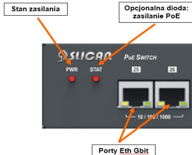
Ilustracja 4.23.: NCP-SWS24 – switch 24 portowy
