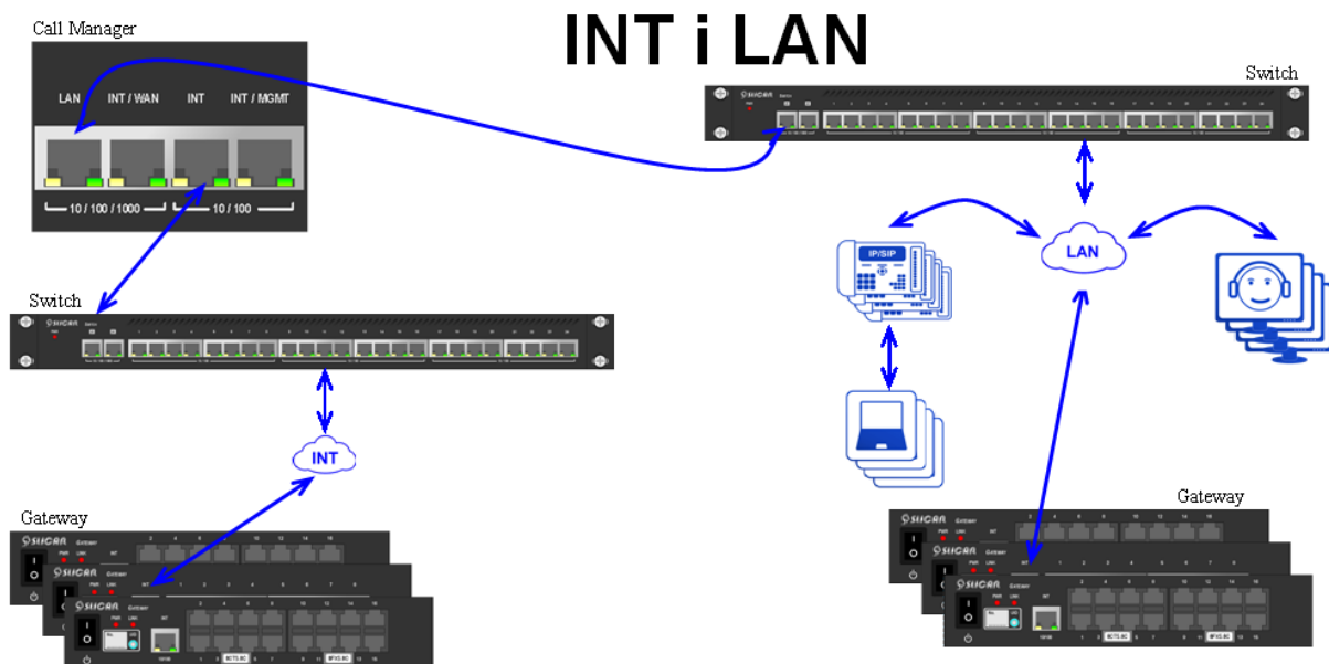
Ilustracja 3.3.: Przykładowa konfiguracja w sieci mieszanej
