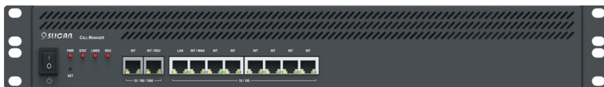
Ilustracja 4.5.: NCP-CM600P – widok z przodu
