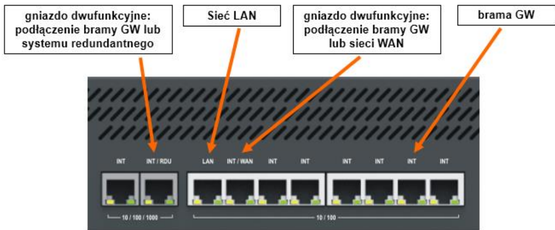
Ilustracja 4.8.: NCP-CM – wbudowany switch
