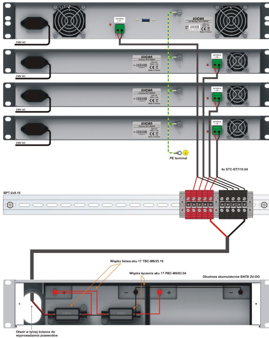
Ilustracja 7.2.: Przyłączenie urządzeń z wykorzystaniem listwy BPT
