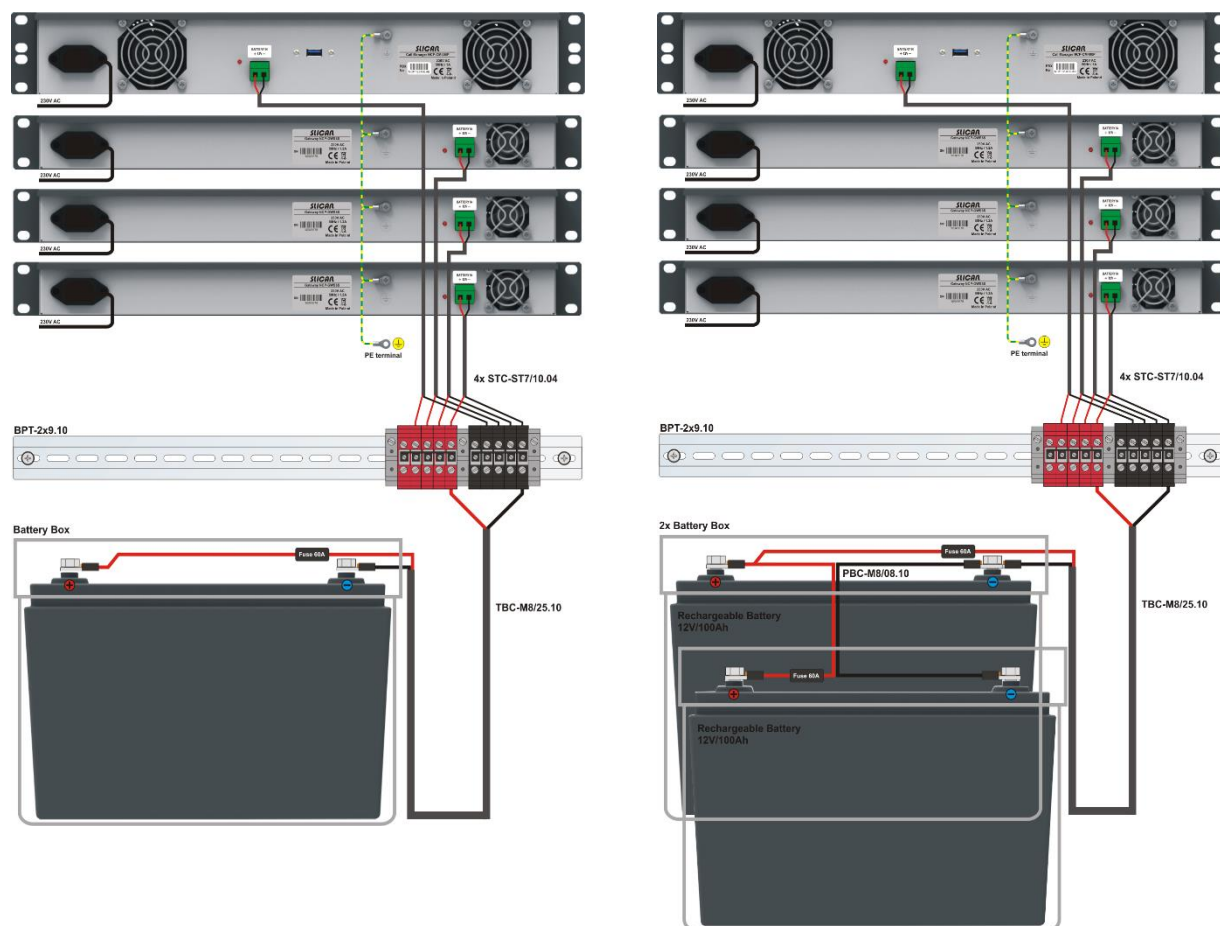
Ilustracja 7.3.: Wykorzystanie listwy BPT i akumulatorów 100Ah
