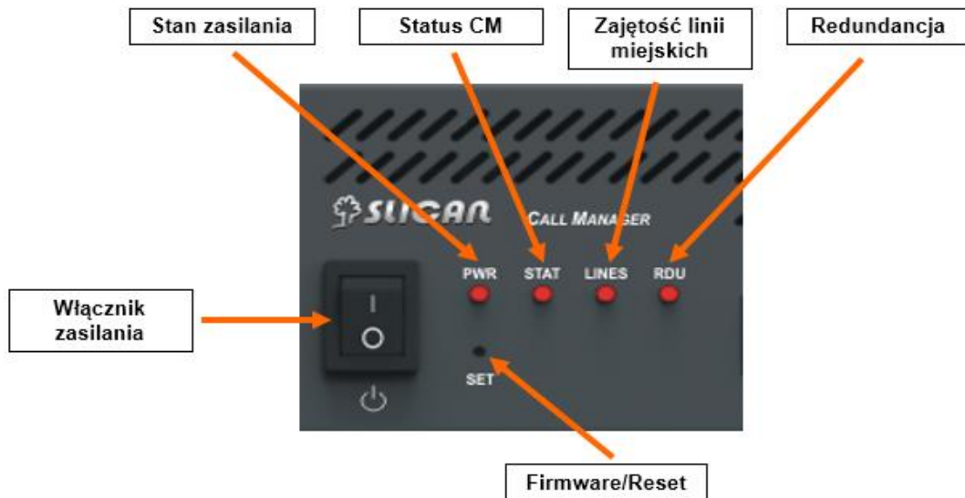
Ilustracja 4.7.: NCP-CM– zespół wskaźników
