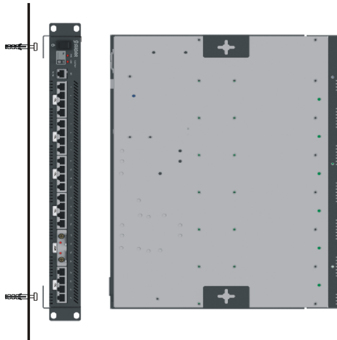
Ilustracja 6.2.: Zastosowanie wieszaka obudowy
