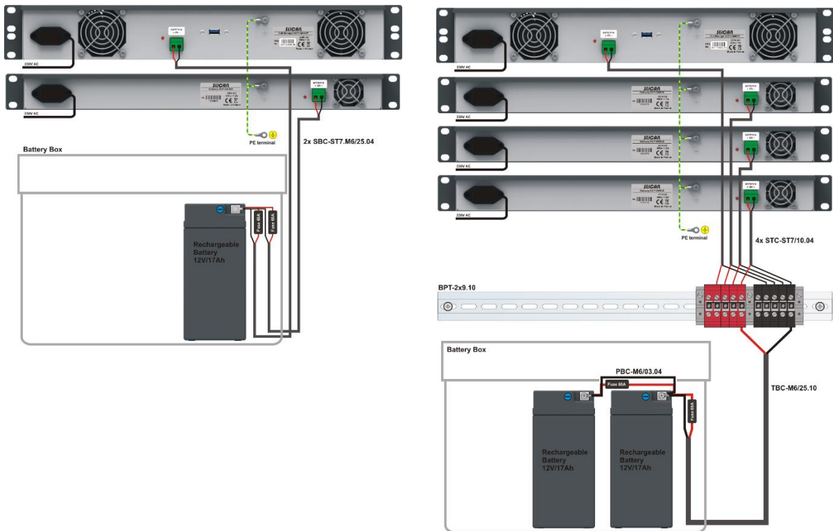
Ilustracja 7.2.: Wykorzystanie akumulatorów 17Ah
