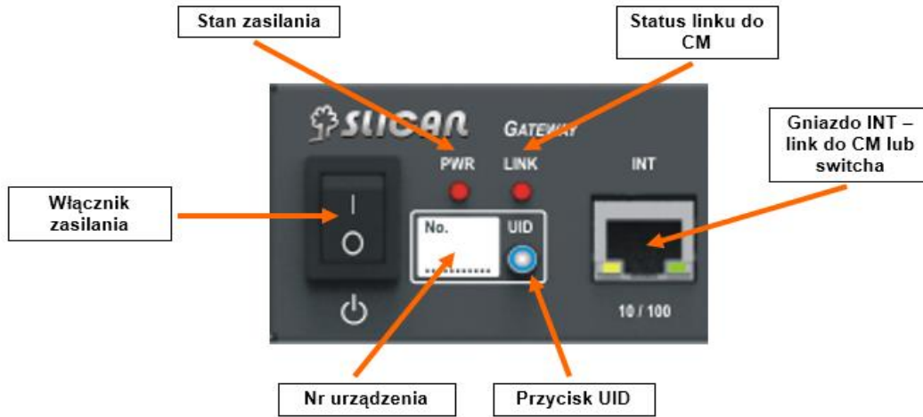
Ilustracja 4.17.: NCP-GW – zespół wskaźników
