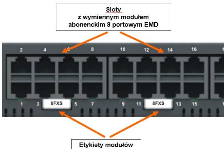
Ilustracja 4.19.: NCP-GWD – wersja z modułami 8 portowymi
