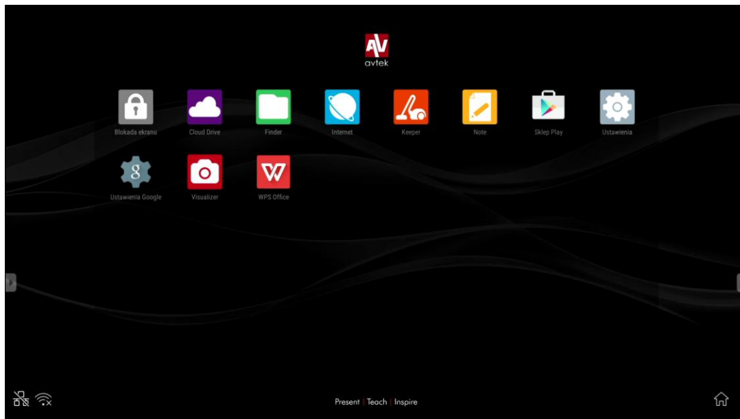
Rys. 1-2 Aplikacje
