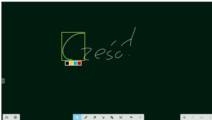
Rys. 3-3-1 Zaznaczanie obiektów
