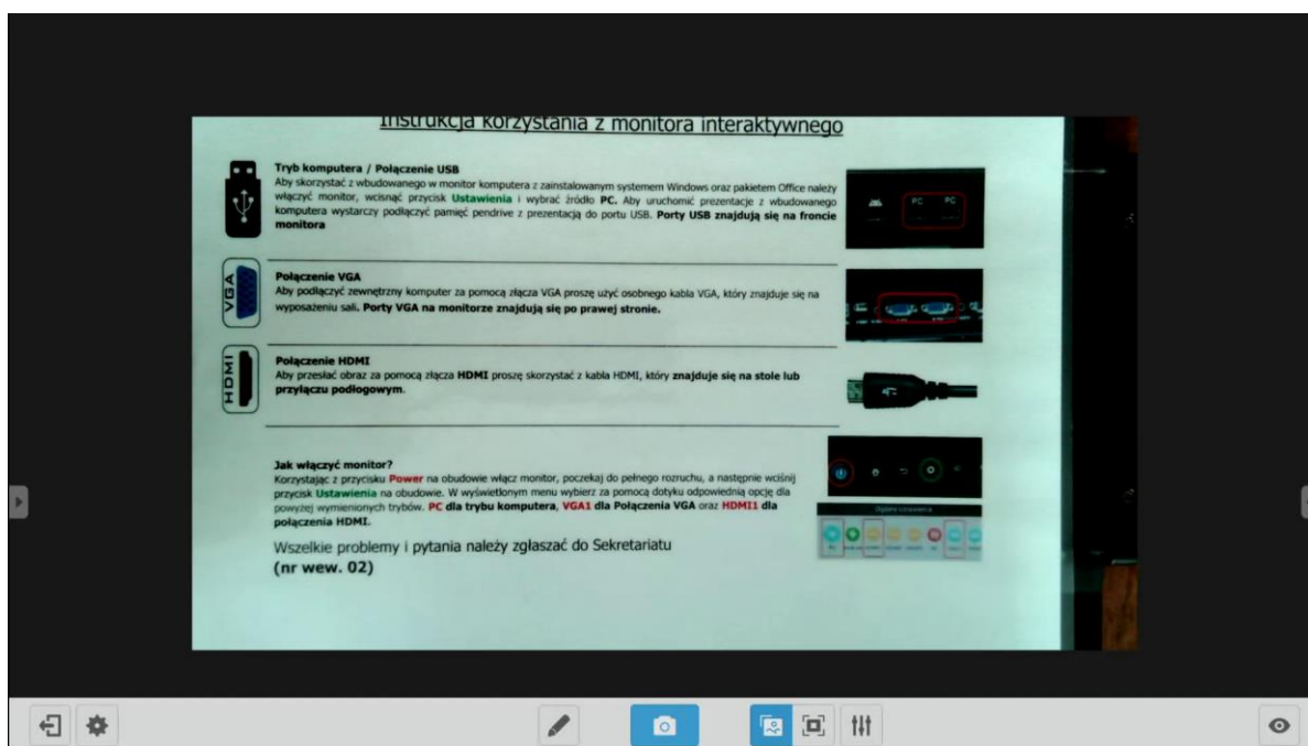
Rys. 5-1 Aplikacja Visualizer
